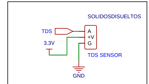
SENSOR DE SÓLIDOS DISUELTOS TDS
