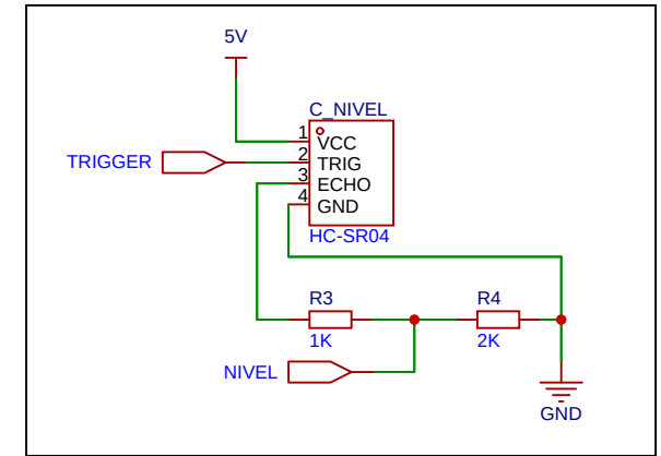
SENSOR DE CONTROL DE NIVEL HC-SR04
