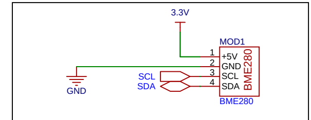
SENSOR DE PRESIÓN, TEMPERATURA Y HUMEDAD BME280
