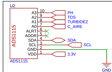
CONVERTIDOR ANALÓGICO DIGITAL ADS1115
